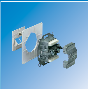
Anschlusskomponenten Datentechnik Csatlakozó eszközök adatátvitelhez
